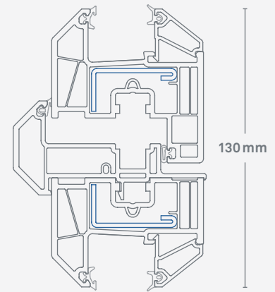
Elite / Stulpausführung Abb.: 1:2,5
